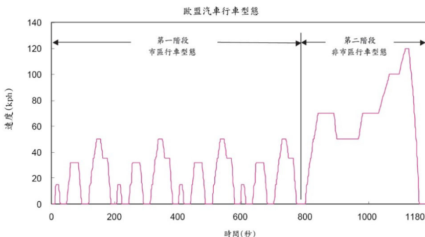
圖三、歐盟 1999/100/EC 指令及其後續修正指令 NEDC 測試程序之行車型態
