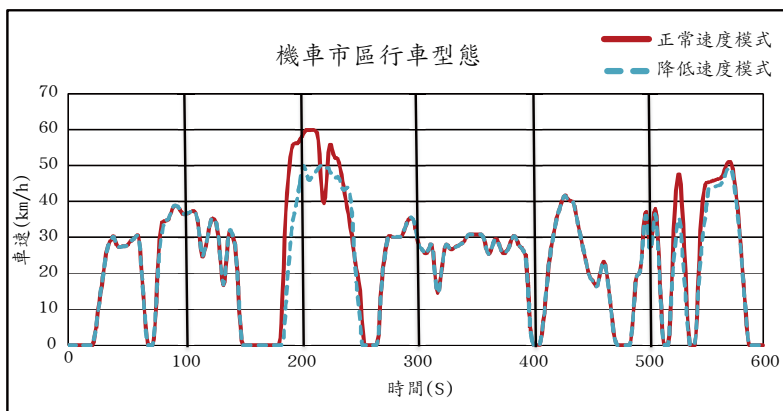
圖四、機車市區行車型態(適用行政院環境保護署「交通工具空氣污染物排放標準」中華民國一百零六年一月一日以後污染排放標準機車。)
