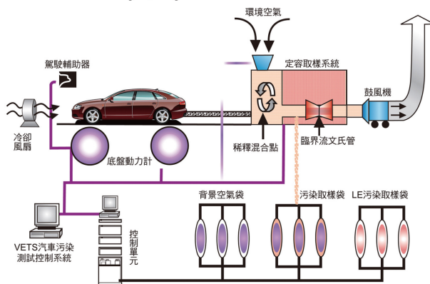
車輛燃油效率及污染測試實驗室相關設備示意圖
