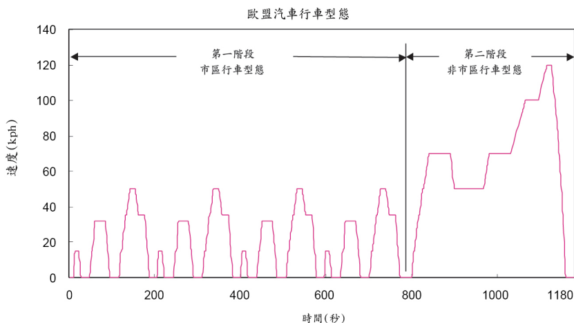
圖三、歐盟1999/100/EC指令及其後續修正指令測試程序之行車型態
